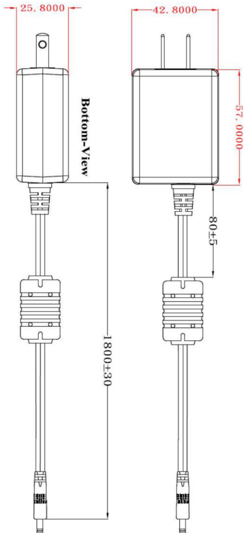
【TWS005W051 外形图】
